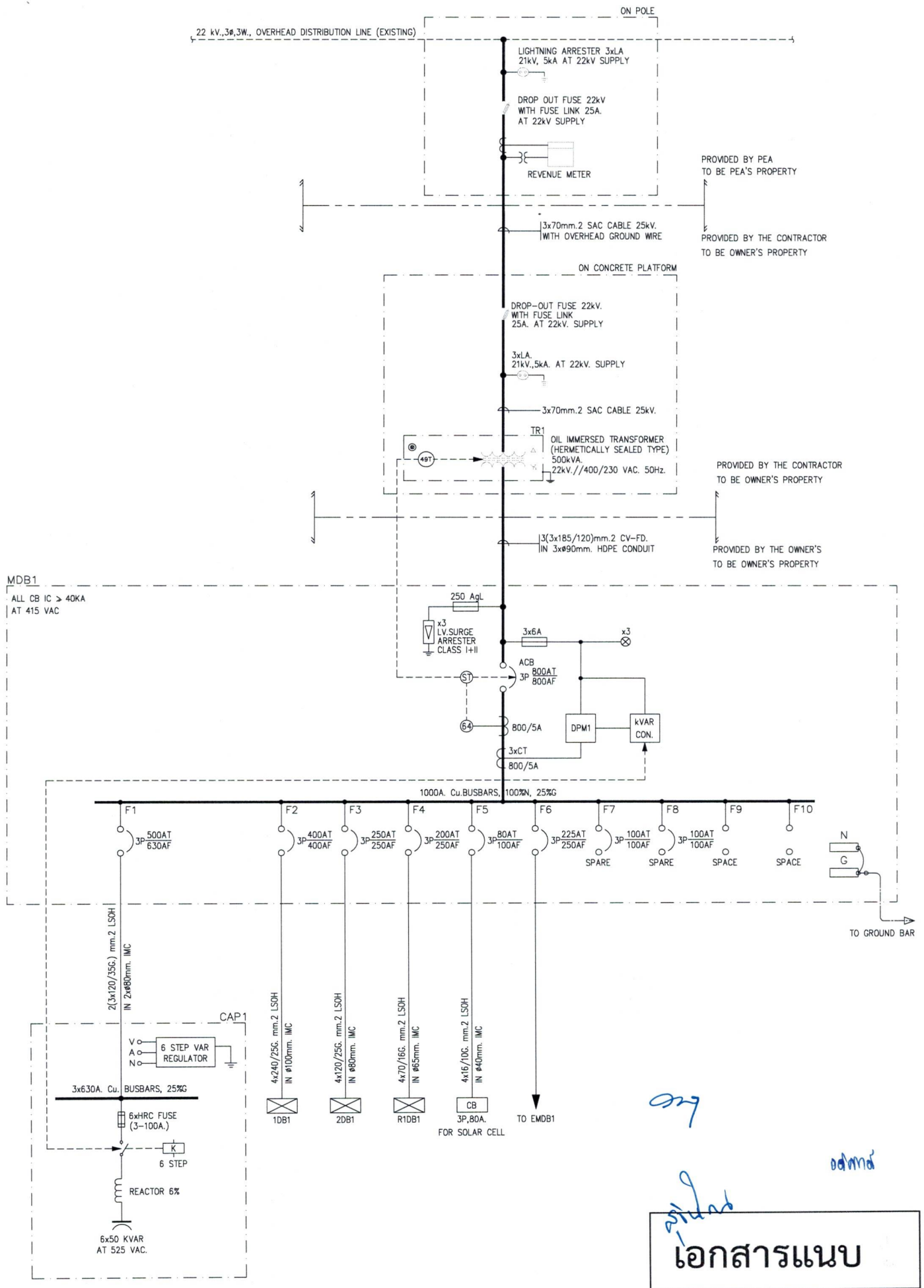
ไดอะแกรมระบบไฟฟ้า 1
