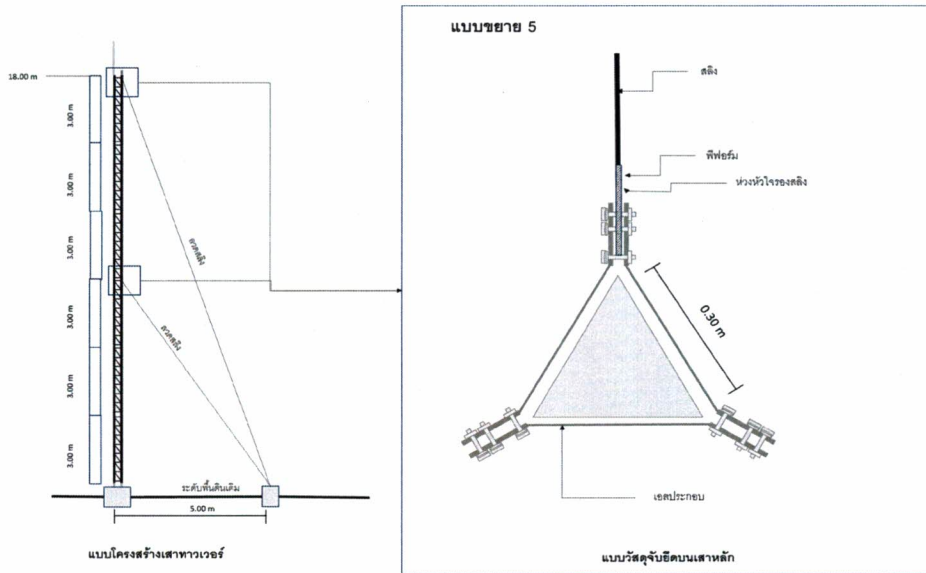
ภาพที่ 7 จัดหาและติดตั้งวัสดุสำหรับจับยึดบนเสาทาวเวอร์
