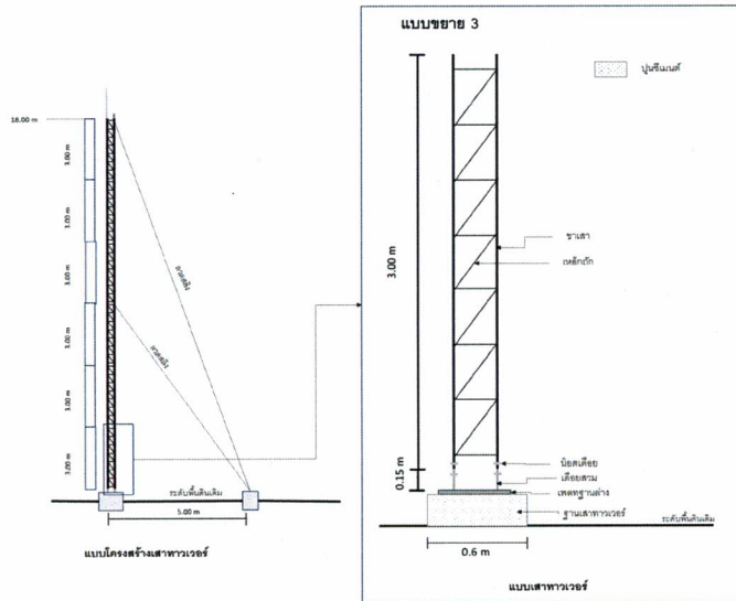
ภาพที่ 5 โครงสร้างเสาทาวเวอร์
