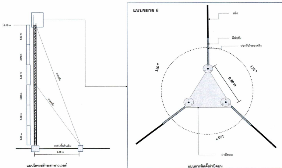
ภาพที่ 8 ติดตั้งวัสดุสำหรับปิดฝานทาวเวอร์
