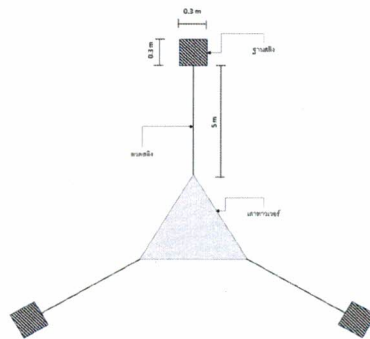
ภาพที่ 2 แบบโครงสร้างเสาทาวเวอร์และฐานสลิงในมุมมองด้านบน
