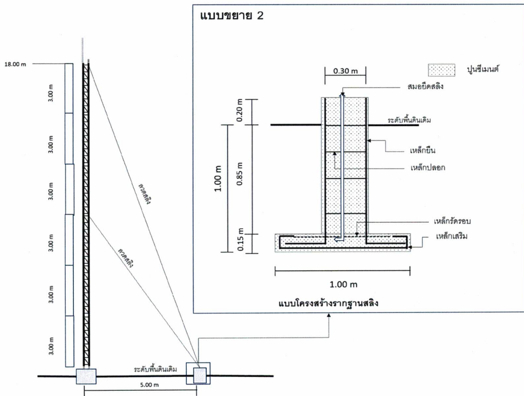
ภาพที่ 4 แบบโครงสร้างรากฐานสลิง
