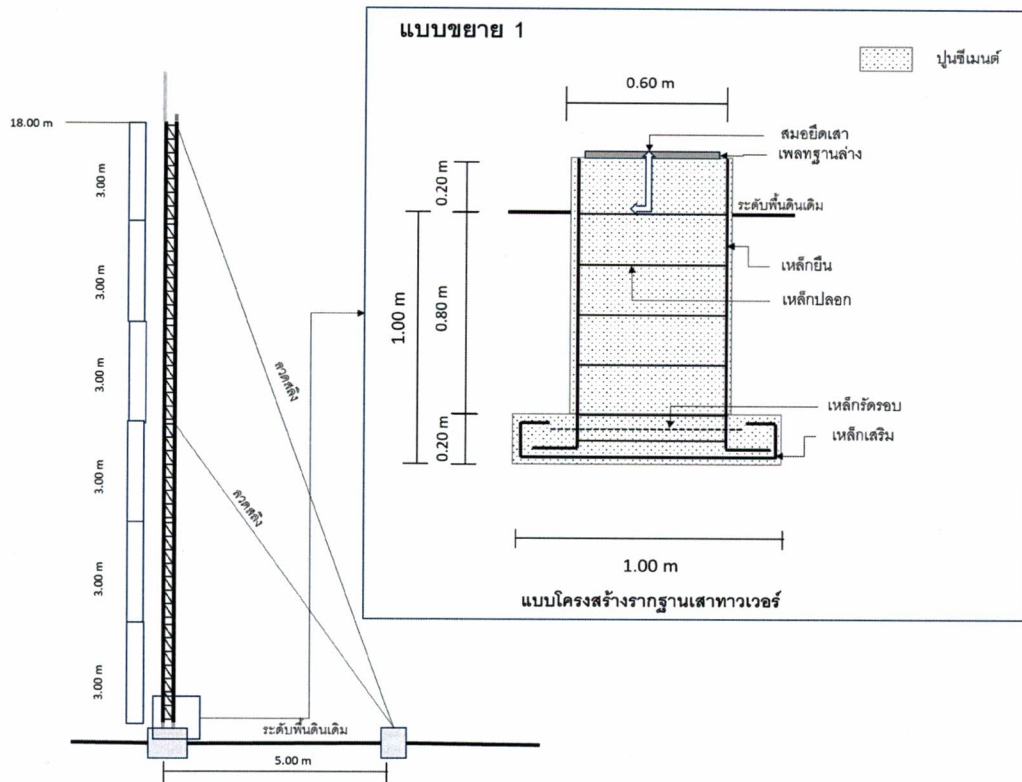
ภาพที่ 3 แบบโครงสร้างรากฐานเสาทาวเวอร์
