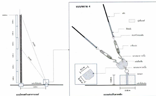
ภาพที่ 6 ติดตั้งวัสดุสำหรับจับยึดเสาทาวเวอร์
