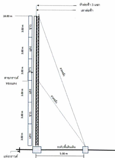
ภาพที่ 1 แบบโครงสร้างเสาทาวเวอร์และระบบล่อฟ้า
