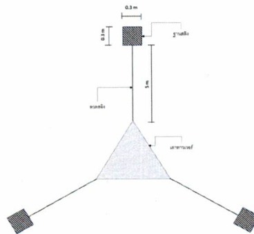
ภาพที่ 2 แบบโครงสร้างเสาทาทาวเวอร์และฐานสลิงในมุมมองด้านบน
