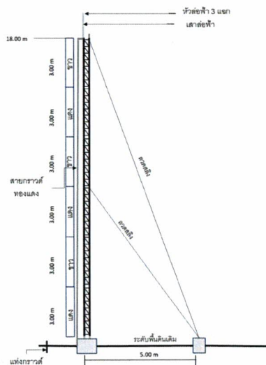
ภาพที่ 1 แบบโครงสร้างเสาทาทาวเวอร์และระบบล่อฟ้า
