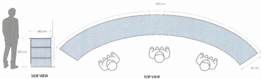
ภาพที่ 2 ภาพแบบในการจัดทำชั้นวางชิ้นงานแบบโค้ง
