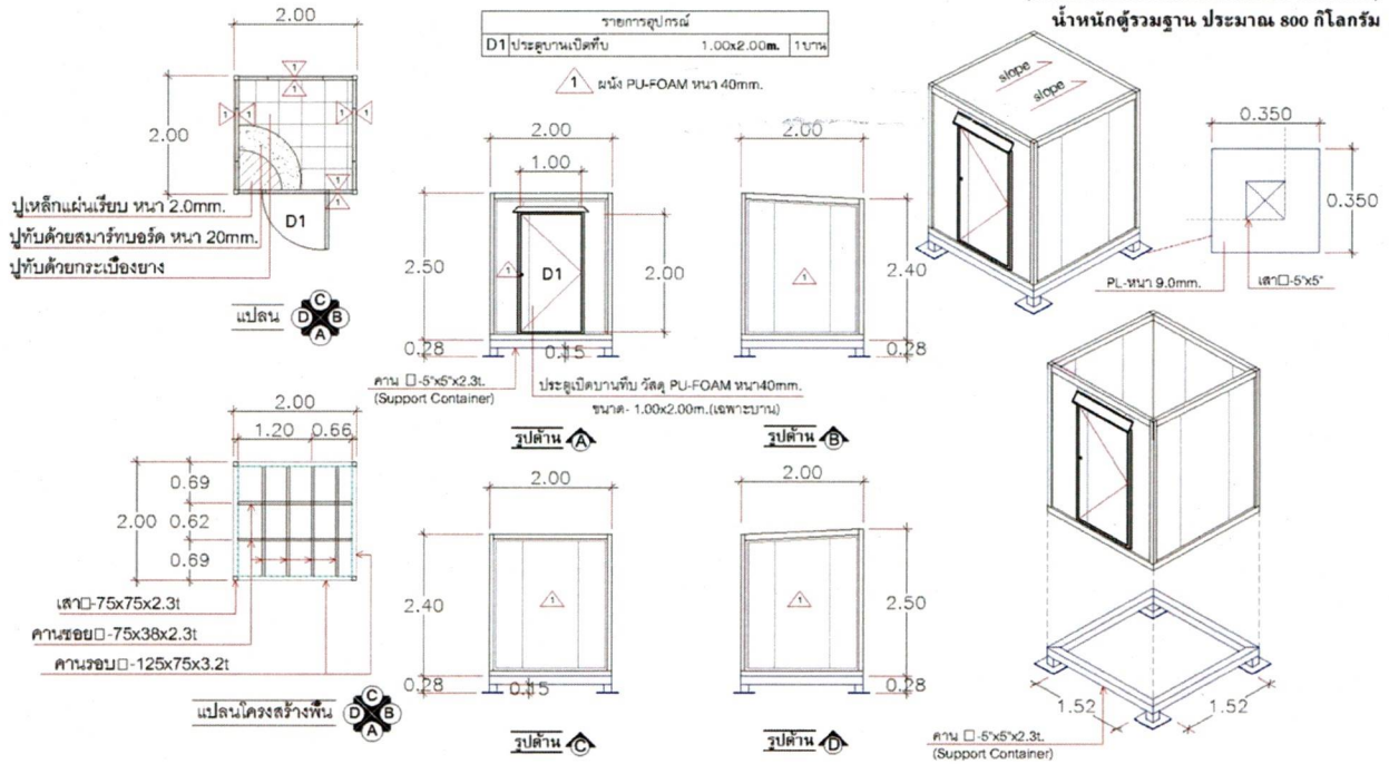
รูปที่ 1 แพลนโครงสร้างครอบเครื่องตรวจวัดอากาศ
