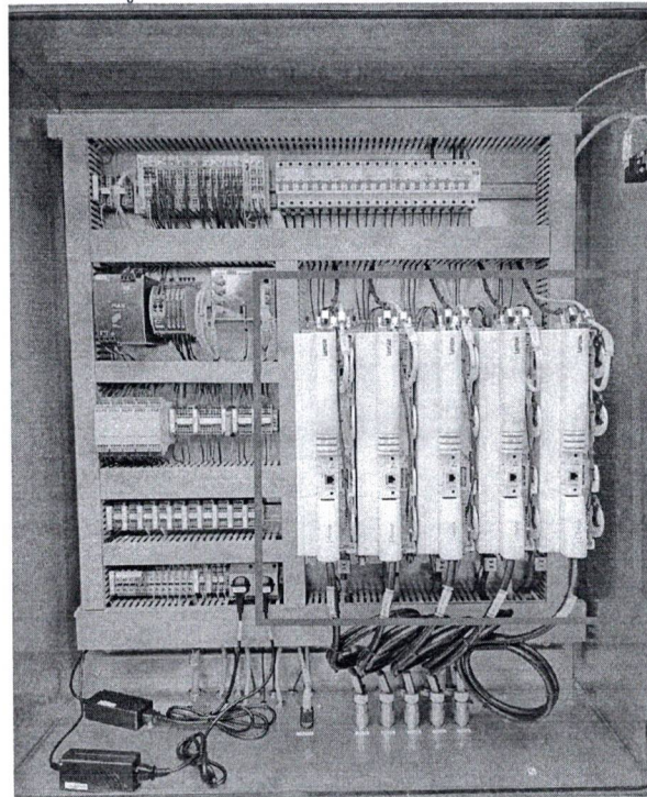
รูปไดร์เวอร์มอเตอร์สำหรับมอเตอร์ M3
