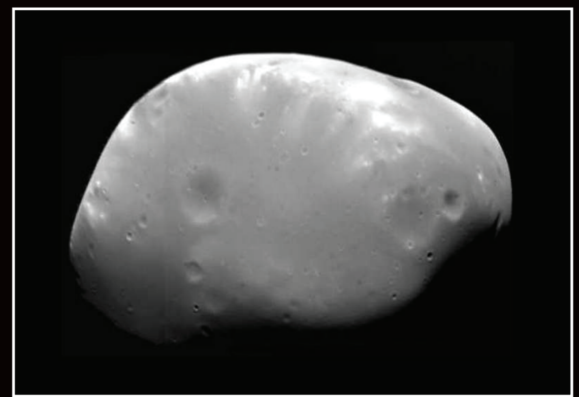
ดวงจันทร์ไดมอส เป็นดวงจันทร์บริวารของดาวอังคารที่มีขนาดเล็ก อยู่ห่างจากดาวอังคารประมาณ 23,400 กิโลเมตร คาบการโคจรรอบดาวอังคาร 30 ชั่วโมง 18 นาที คาบการโคจรรอบดาวอังคาร 7 ชั่วโมง 39 นาที
