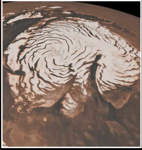
ภาพน้ำแข็งบริเวณ ขั้วเหนือของดาวอังคาร
