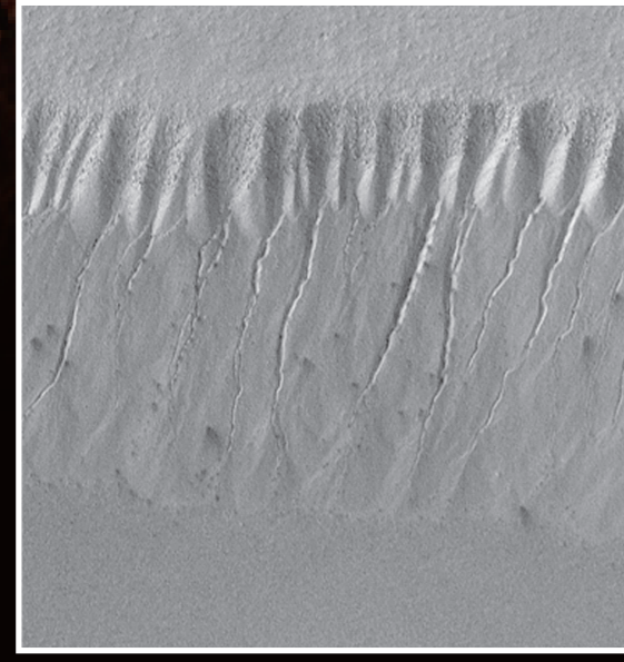
ร่องรอยที่เกิดจาก น้ำไหลในอดีต
