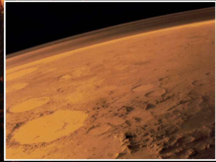
ชั้นบรรยากาศสีส้มบางเบา ปกคลุมผิวดาวอังคาร
