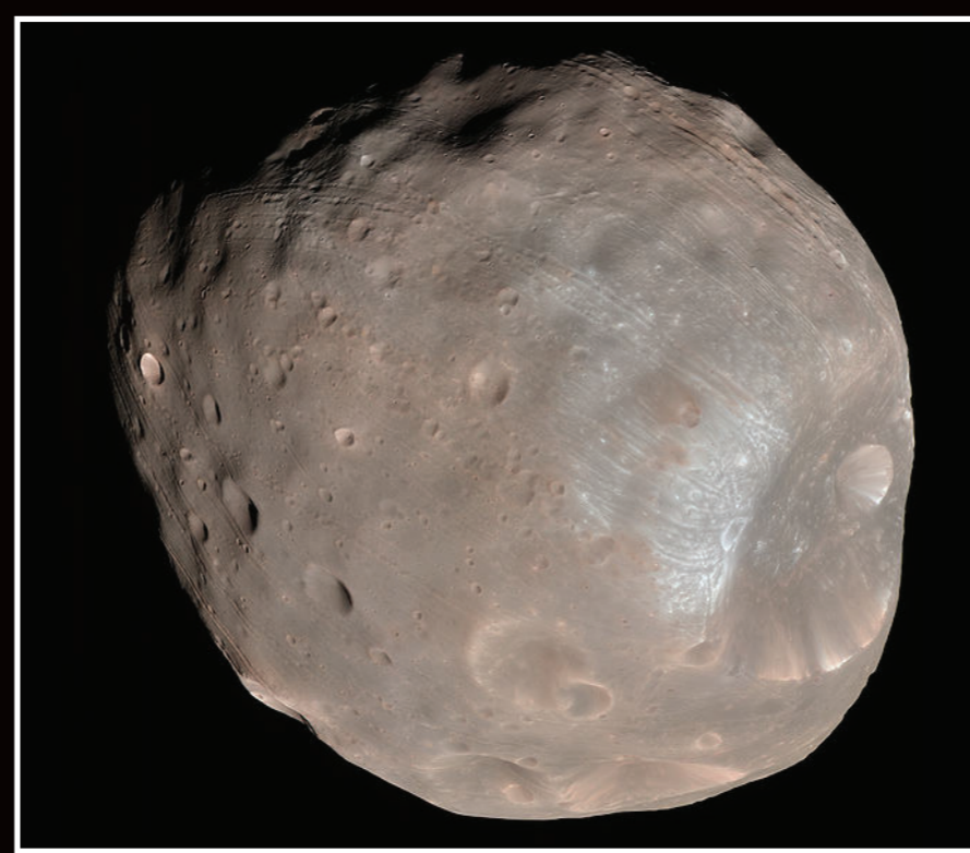
ดวงจันทร์โฟบอส เป็นดวงจันทร์บริวารที่อยู่ใกล้ดาวอังคารมากที่สุด ประมาณ 9,300 กิโลเมตร มีรูปร่างเหมือนมันฝรั่ง ขนาดประมาณ 20 กิโลเมตร คาบการโคจรรอบดาวอังคาร 7 ชั่วโมง 39 นาที
